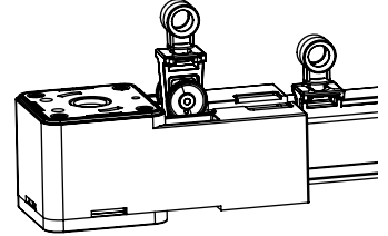
RIPPLEFOLD
