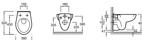
NF E4345-00 Brive - Cuvette suspendue 52 x 36 cm. Fonctionnement basse consommation double chasse 2,6/4 L ou 3/6 L.
