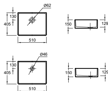
NF ESA01-00 Delta - Timbre à poser 50 x 40 cm sans trop plein, émaillé 3 faces pour une installation adossée au mur. Vidage recommandé: Bonde à grille 62 mm E78561.
