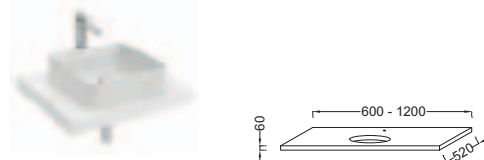
Plan avec 1 découpe pour vasques à poser Vox EVF102 et EVG102 L 600 x P 520 mm – stratifié* EB60-0600 – bois massif** EI00-0600 L 800 x P 520 mm – stratifié* EB62-0800 – bois massif** EI01-0800 L 1000 x P 520 mm – stratifié* EB64-1000 – bois massif** EI02-1000 L 1200 x P 520 mm – stratifié* EB66-1200 – bois massif** EI03-1200 Stratifié à partir de 309 € TTC – Bois massif à partir de 589 € TTC dont 1 € d'éco-participation
