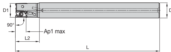
Reduzierter Schaft
