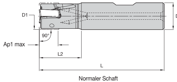
Normaler Schaft
