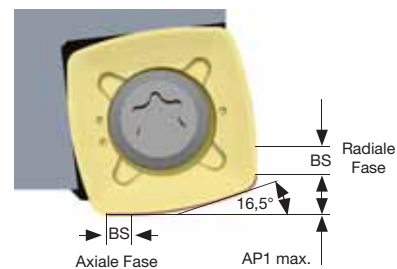
Perfekte Kombination aus runden und quadratischen Wendeschneidplatten-Baureihen.
