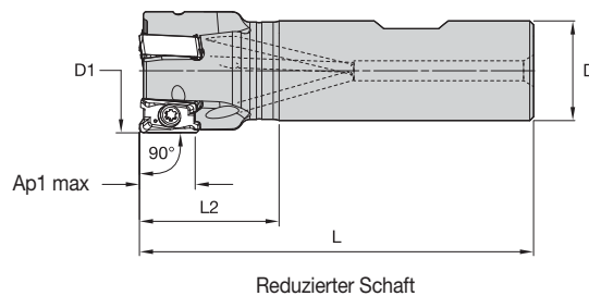
Reduzierter Schaft
