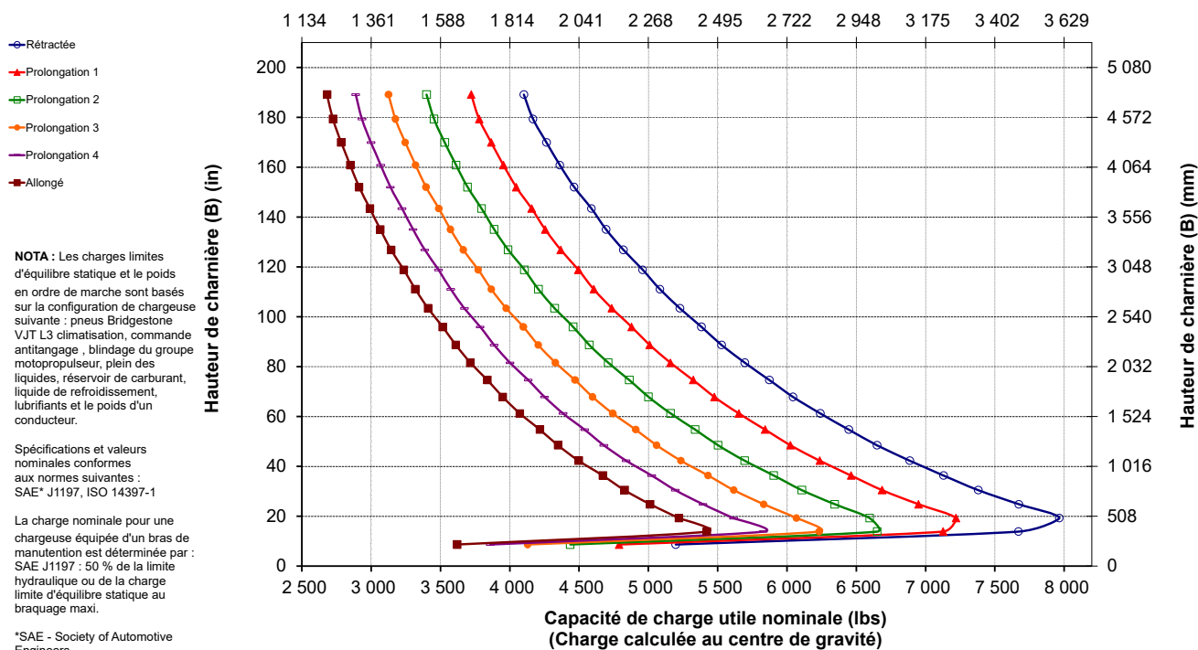
Capacité de charge utile nominale (kg) (Charge calculée au centre de gravité)
