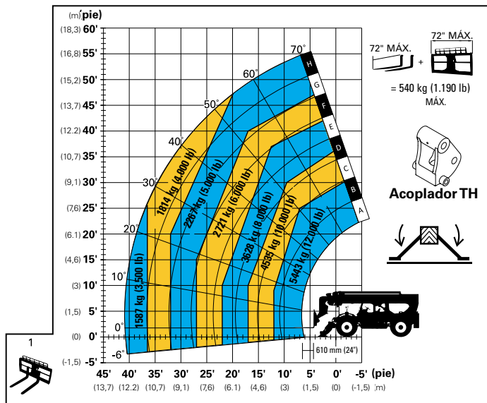
Estabilizadores bajados
