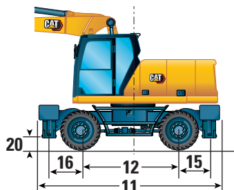
Podwozie z 2 zestawami podpór
