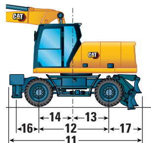
Podwozie z 1 zestawem podpór i lemieszem
