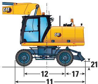
Podwozie z samym lemieszem
