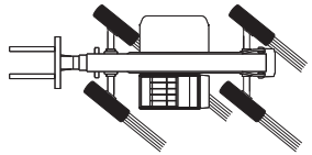
STERZATA LATERALE A 4 RUOTE
