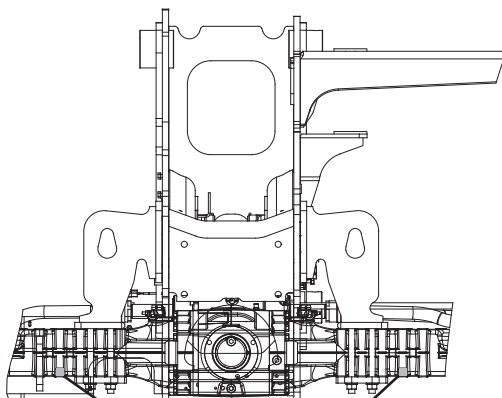
VEDEREA C-C
