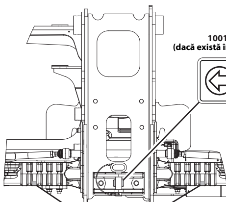
VEDEREA D-D
