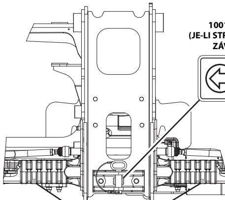
POHLED D-D
