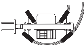
4-КОЛЕСНО КРЪГОВО КОРМИЛНО УПРАВЛЕНИЕ
