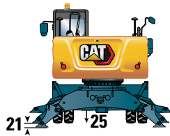
Tren de rodaje con 2 juegos de estabilizadores
