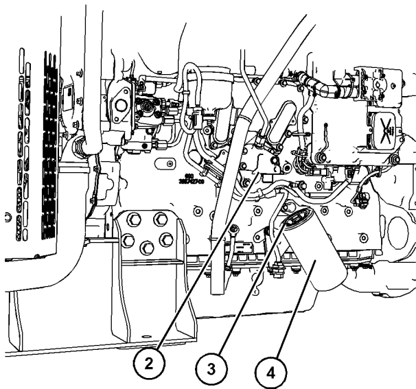
图 47 g06279035 典型示例
