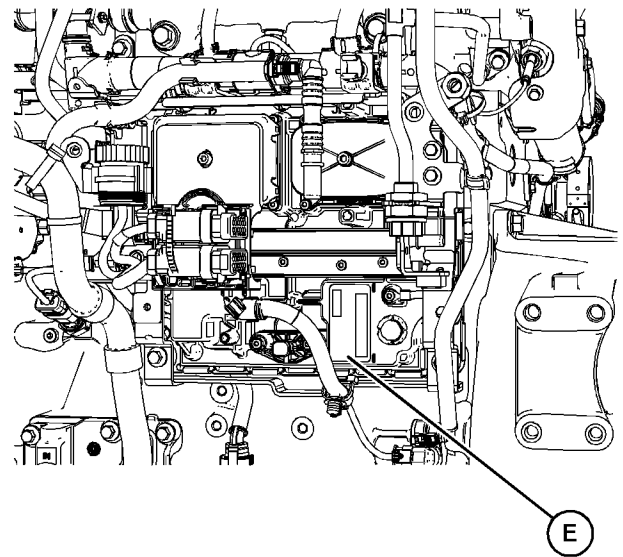
图 25 典型示例 (E) ECM 标志的位置 g07116056
