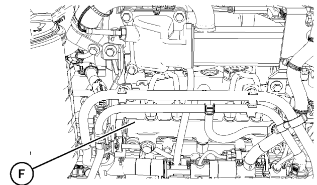
图 26 典型示例 (F) 燃油歧管 (油轨) 标志的位置 g07168783
