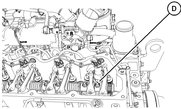
图 24 典型示例 (D) 电子单体喷油器标记的位置 拆下喷油器卡箍，以显示标记位置 g07168768
