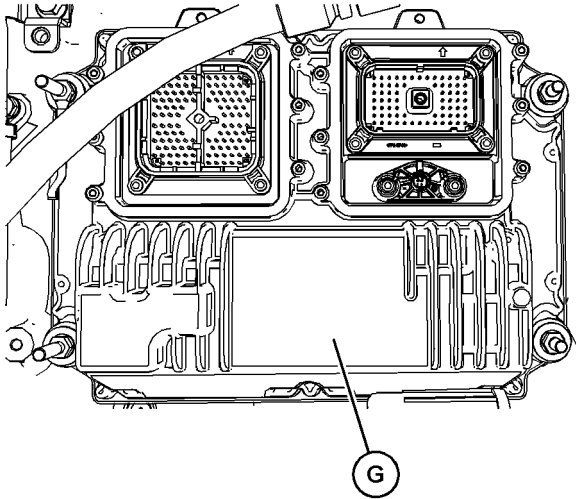
图 23 典型示例 (G) ECM 标志的位置 g06764652
