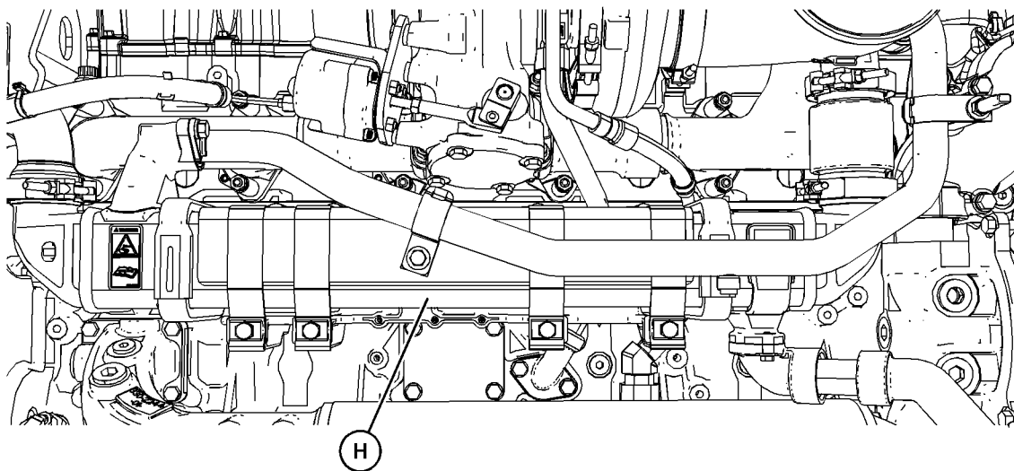
图 24 典型示例 (H) 废气冷却器 (NRS) 标记的位置 i08803809 g06773509
