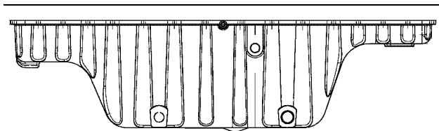
图 63 中间油底壳
