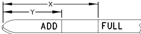
图 92 油尺的部分视图 g00110310
