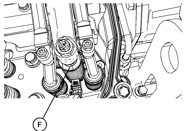
图 22 典型示例 (F) 电子单体喷油器标记的位置
