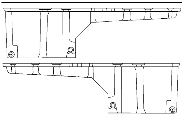
图 62 标准油底壳
