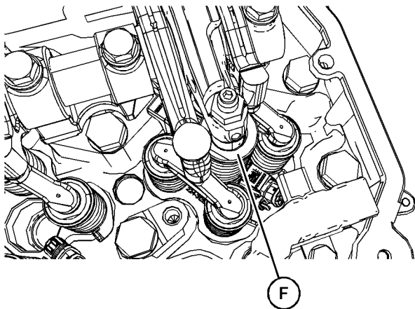
图 28 典型示例 (F) 电子单体喷油器标记的位置 g06764647
