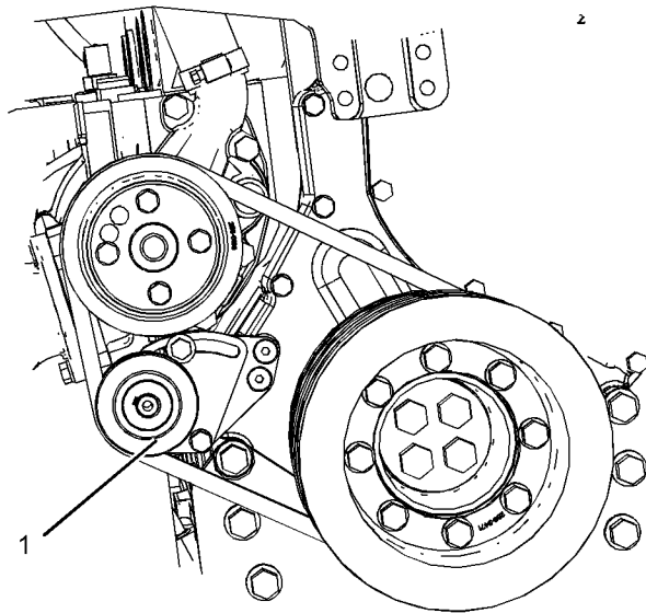
图 77 典型示例 g03748098
