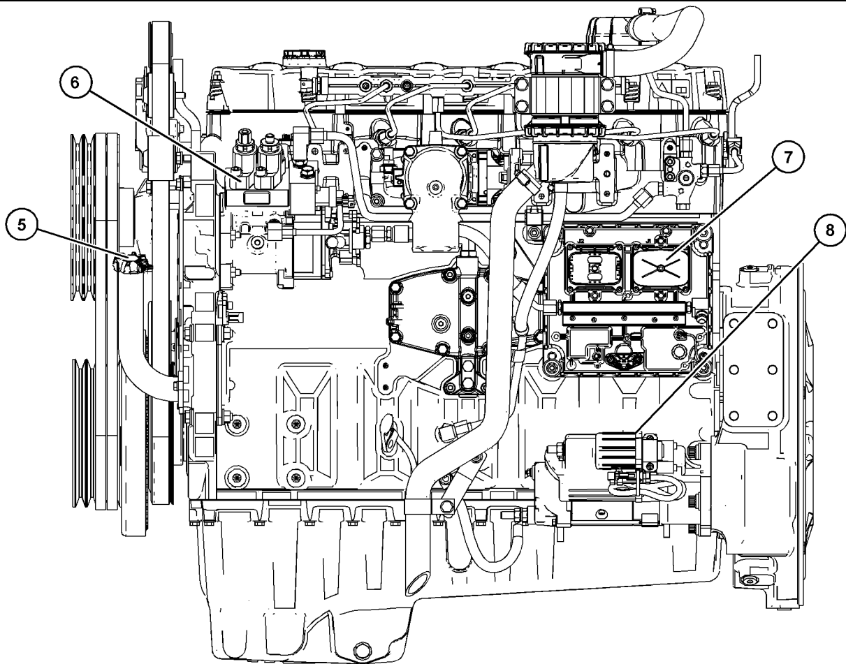
典型发动机左侧视图
