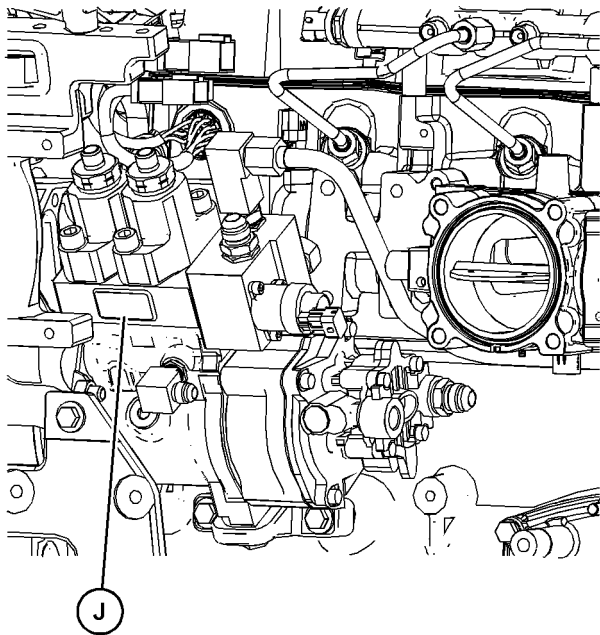
图 31 典型示例 (J) 喷油泵标志的位置
