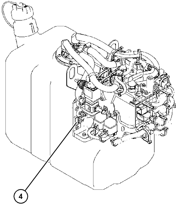
图 38 典型示例 (4) PTU 标牌位置 g06251091
