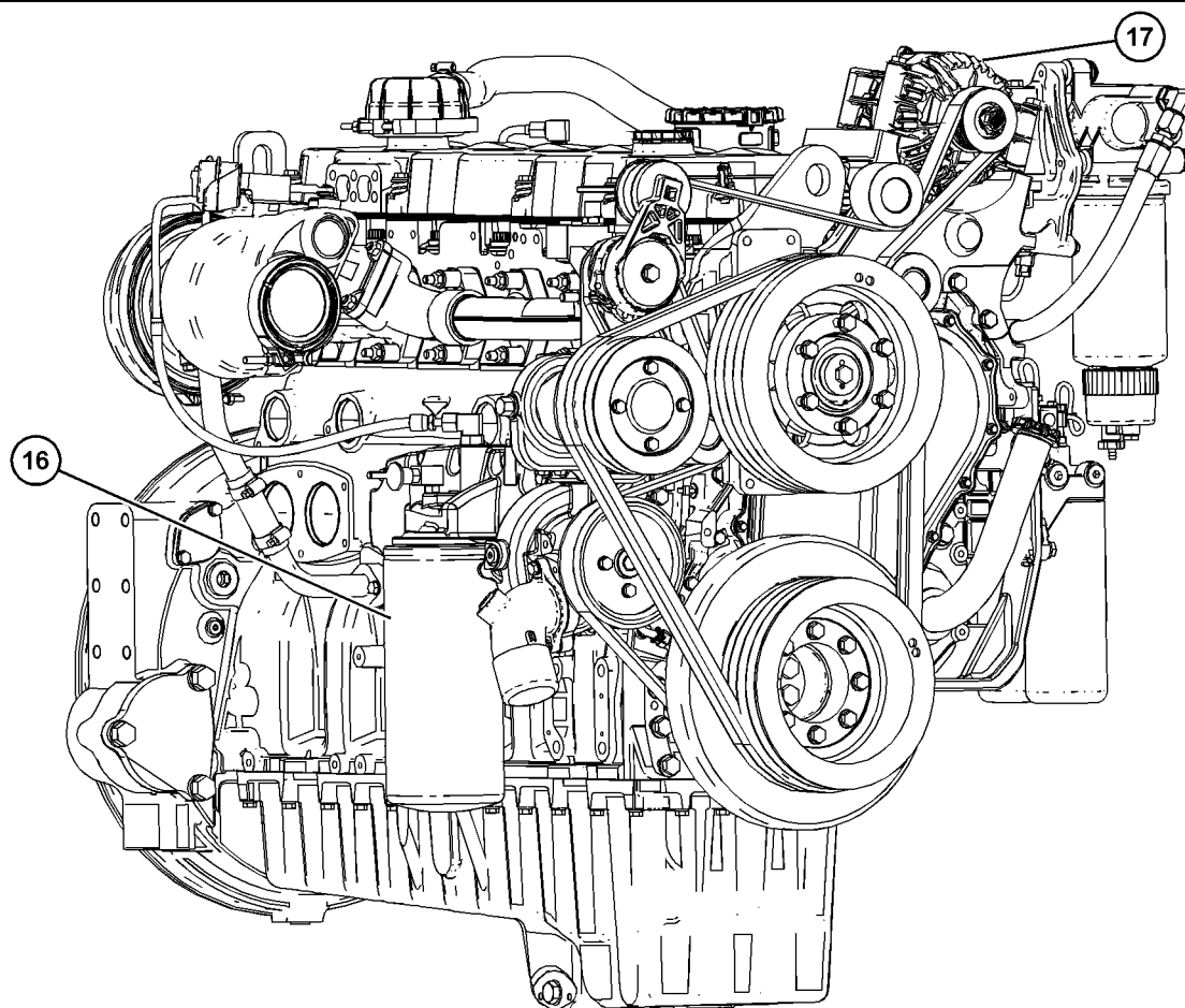
图 21 典型发动机右前侧视图
