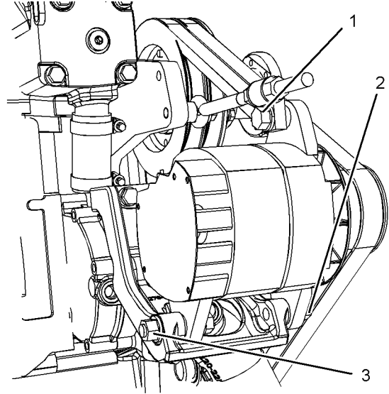
图 78 典型示例 g03748150
