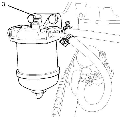
图 52 带滤罐的燃油滤清器 (3) 通风螺钉
