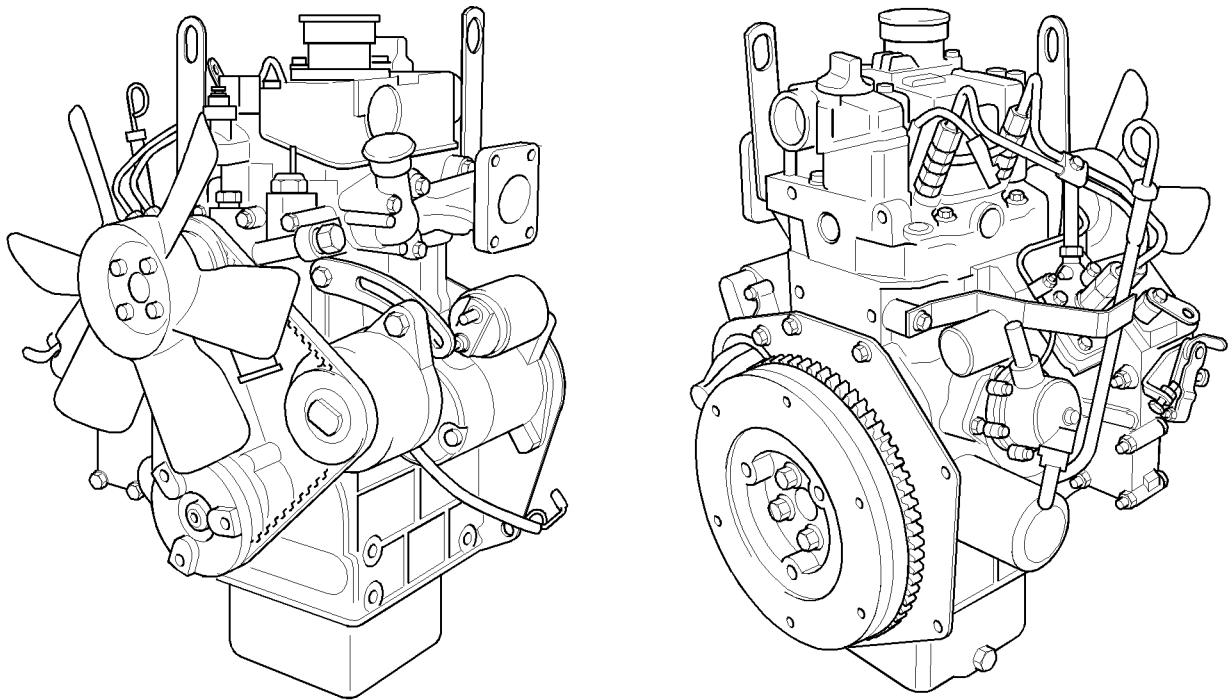
图 11 402C-05 发动机的典型视图
