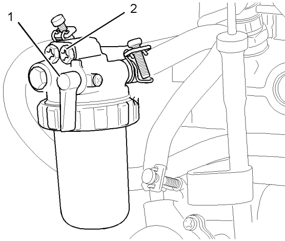
图 51 带滤芯的燃油滤清器 (1) 燃油阀 (2) 通风螺钉
