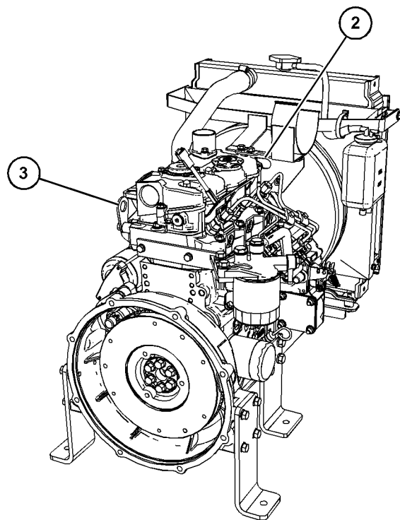
图 28 工业用开放式动力装置 (IOPU 的典型示例 (2) 前吊耳 (3) 后吊耳
