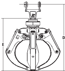
Garfios de 4 dientes
