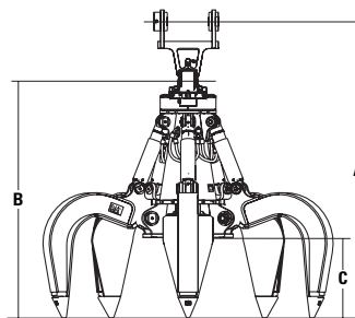
Garfios de 5 dientes
