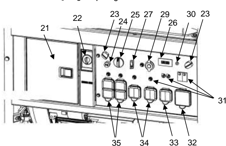
Panneau sans Détecteur de monoxyde de carbone
