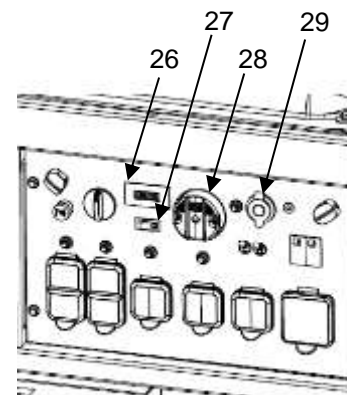
Panneau avec Détecteur de monoxyde de carbone
