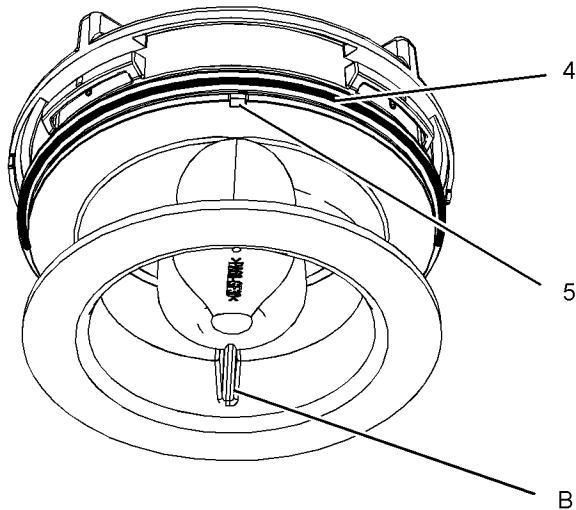
图 64 (B) 对准位置 g01884135
