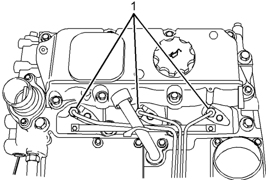
图 38 g01228000 喷油器螺母
