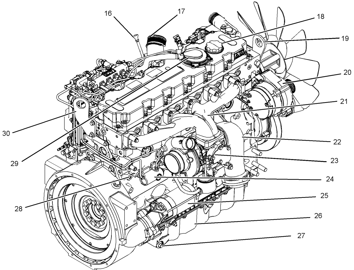
图 19 发动机右后视图
