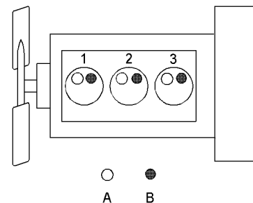
图 12 气门布置的典型示例
