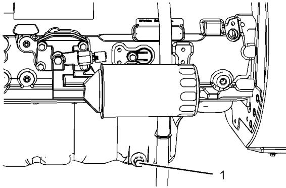
图 31 机油排放塞 g01356033
