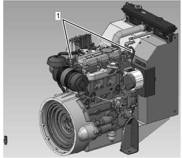
图 25 一些三缸应用中可能安装有吊耳，如图 25 所示。 g03791033 (1) 吊耳
