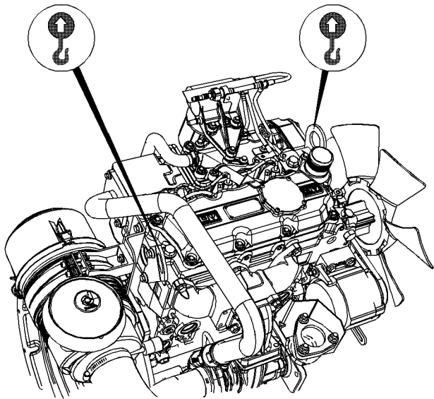
图 24 三个气缸吊耳的典型示例 g03791046
