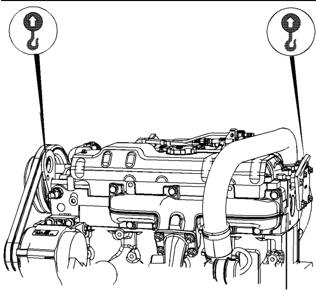
图 23 四个气缸吊耳的典型示例 g03729078
