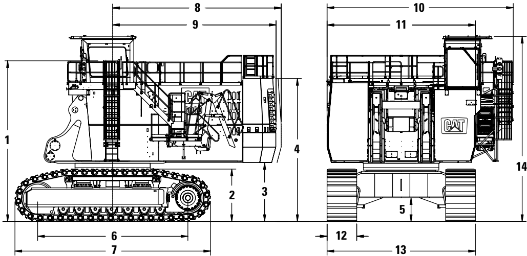
Unité de base 6060/6060 FS
