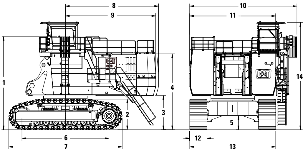
Unité de base 6060 AC/6060 AC FS
