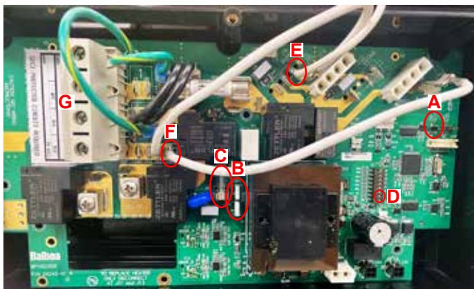
115 Volt Connected
