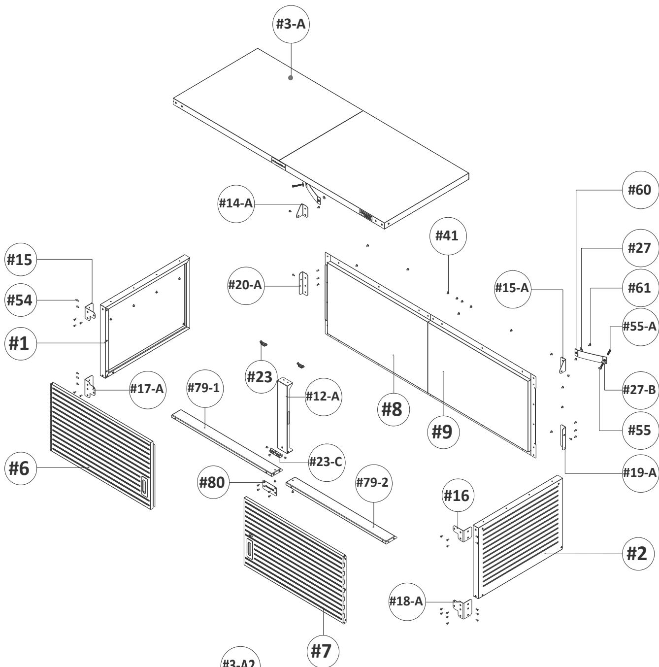
(#3-A) Top Panel
