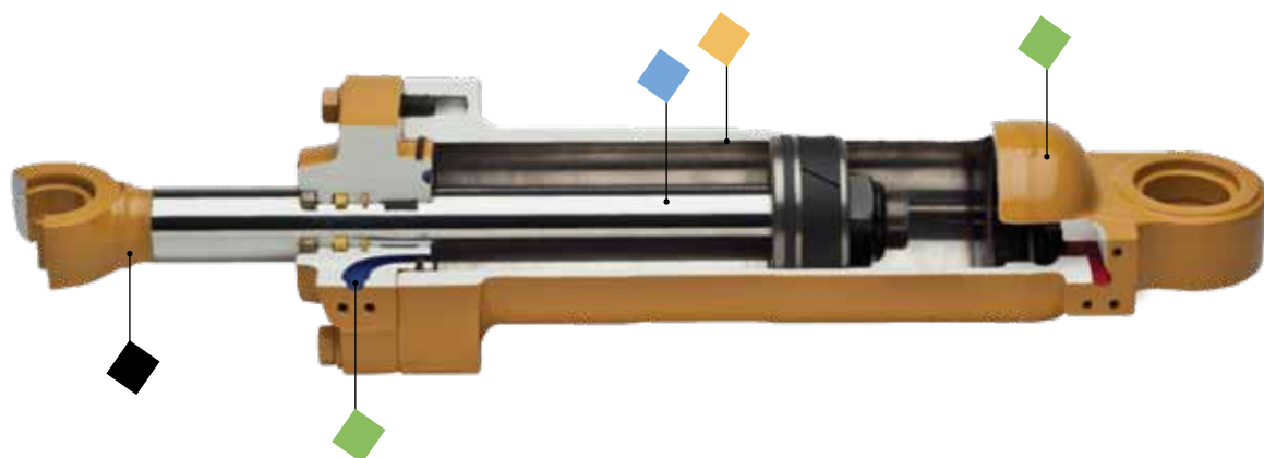
■ STÅNGÖGLA ■ ÄNDSTYCKE OCH TÄTNINGAR ■ KOLVSTÅNG ■ CYLINDERMANTEL
