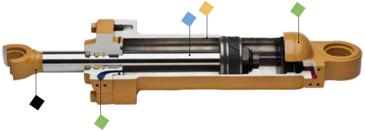
◆ حلقة القضيب ◆ الغطاء الطرفي وموانع التسرب ◆ قضيب الكباس ◆ بدن أنبوب الأسطوانة
