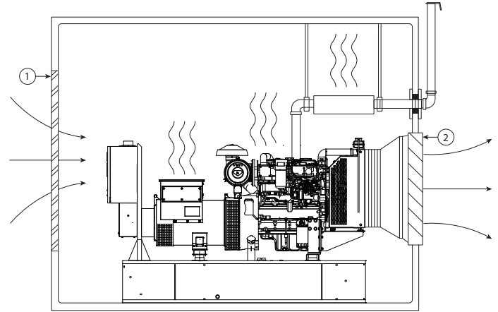
صورة 4.1 - تركيب قياسي يوضح تهوية المولد
