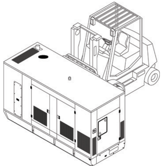
صورة 4.4 – نقل المولد باستخدام ونش بمرفاع شوكي وترولي برافعة شوكية
