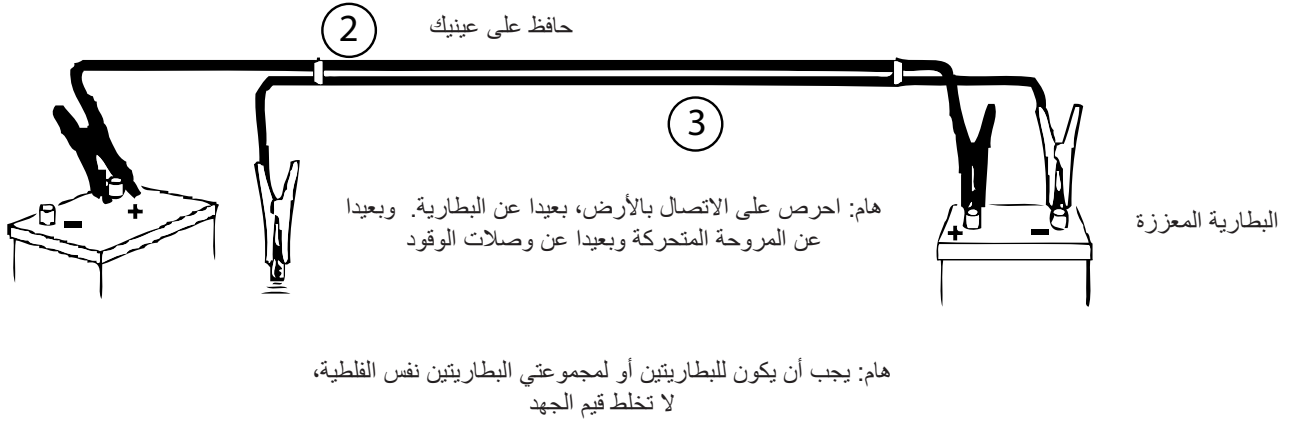
صورة 6.4 - بدء التشغيل باستخدام كابلات بدء التشغيل
