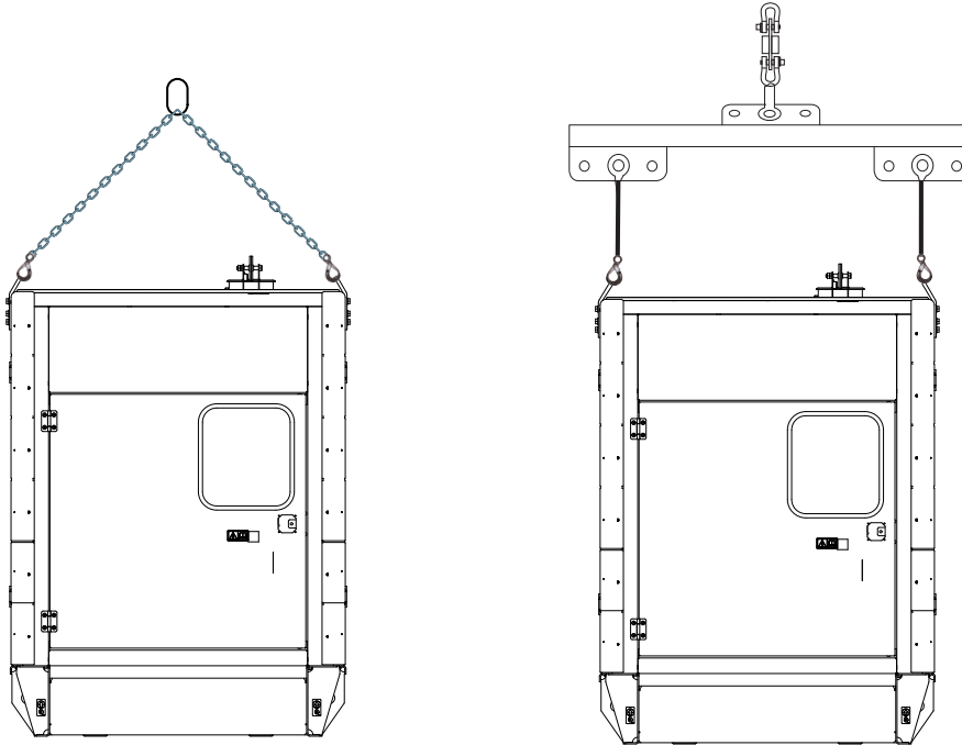
صورة 4.7 – تجهيزه رفع ثنائية النقطة
