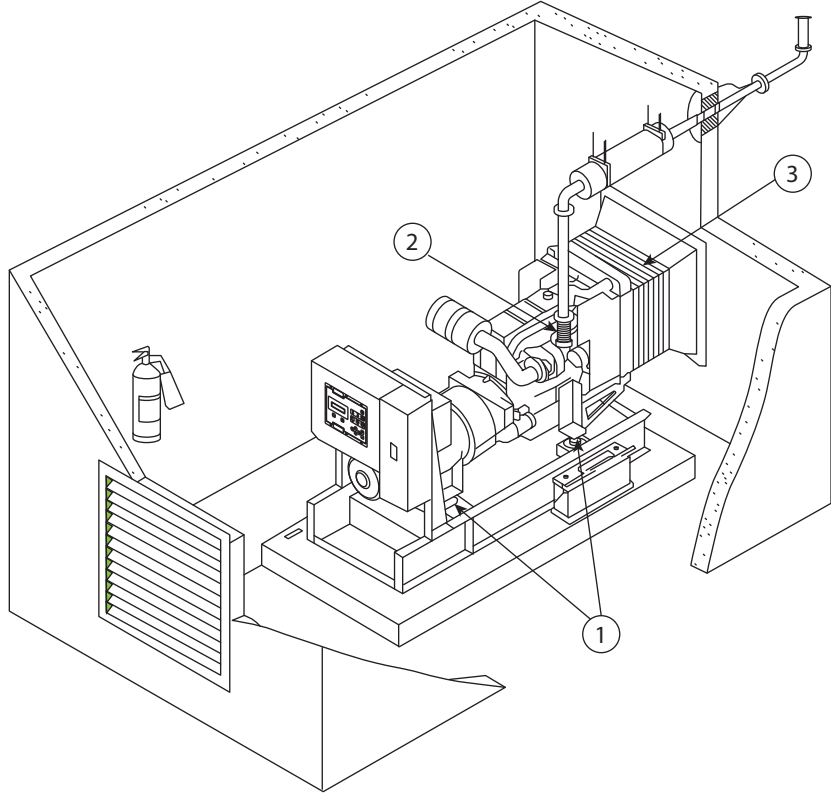
صورة 4.11 - تركيب قياسي يبرز تقنيات تخميد الاهتزازات
