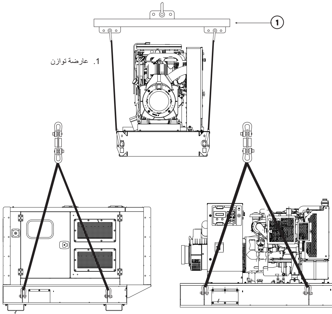
صورة 4.8 – استعدادات الرفع الصحيحة لتركيب المولد الكهربائي (مكشوف أو داخل صندوق)
