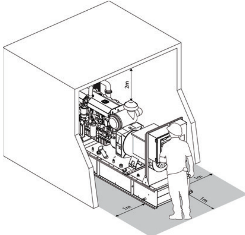
صورة 4.2 - تركيب قياسي يبين المدخل للمولد ومكان عمل المشغل
