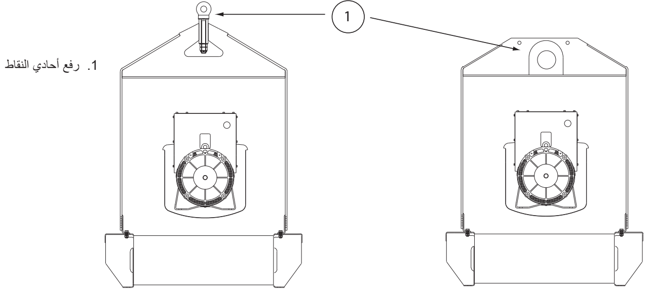
صورة 4.6 – تجهيزه رفع أحادية النقطة
