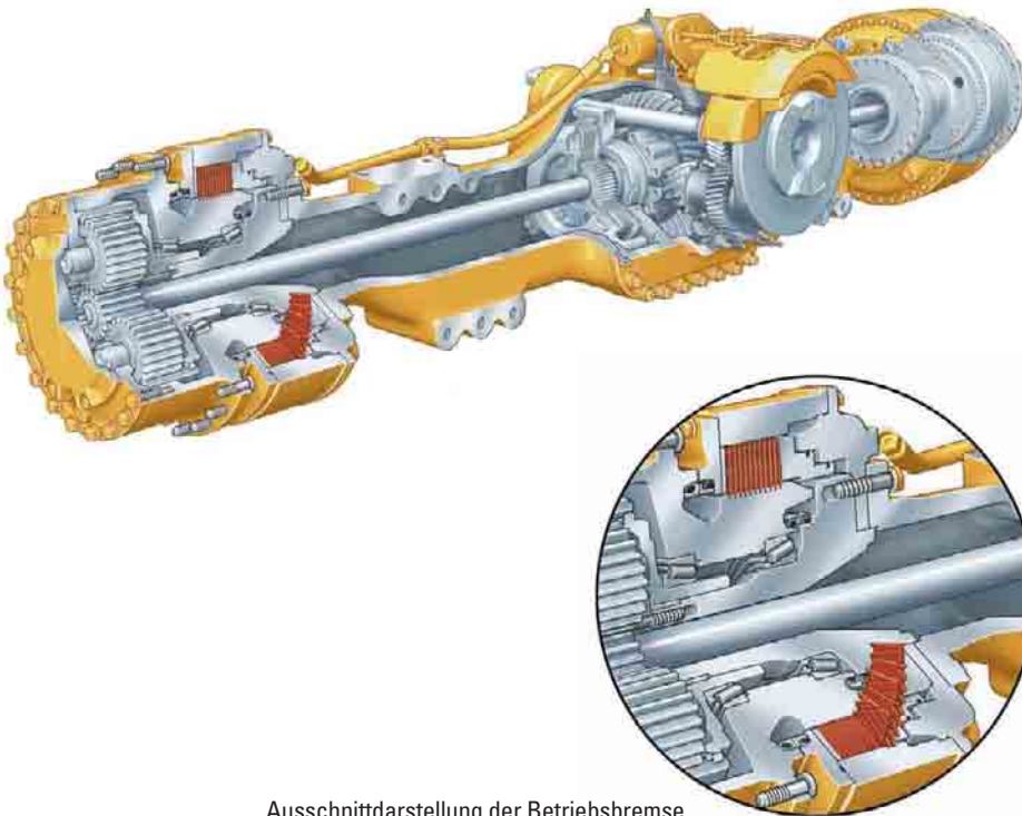
Ausschnittdarstellung der Betriebsbremse
