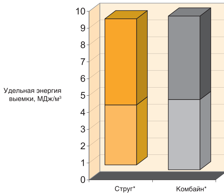
Рис. 11: удельная энергия комбайновых и струговых установок
