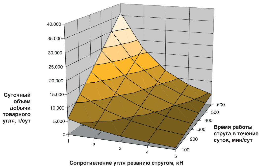
Рис. 13: Производительность струговой установки в зависимости от удельной энергии выемки и суточного времени работы струга
