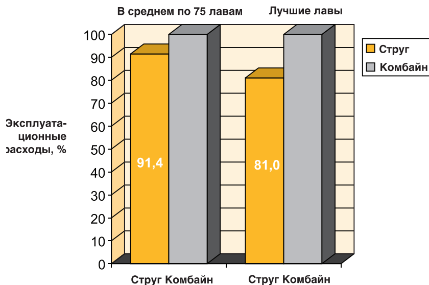
Рис. 16. Сравнение эксплуатационных расходов для комбайновых и струговых лав Германии
