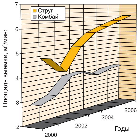
Рис. 7. Средняя площадь выемки в длинных очистных забоях на шахтах Германии 1
