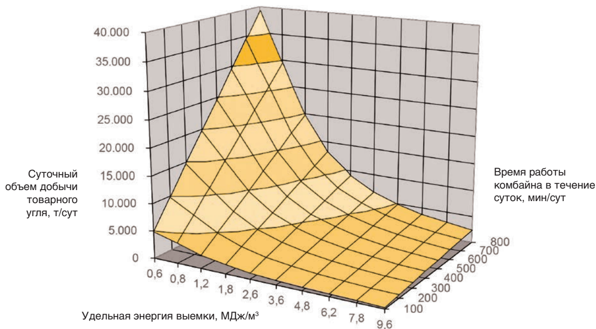
Рис. 12. Производительность комбайновой лавы в зависимости от величины удельной энергии и времени работы комбайна
