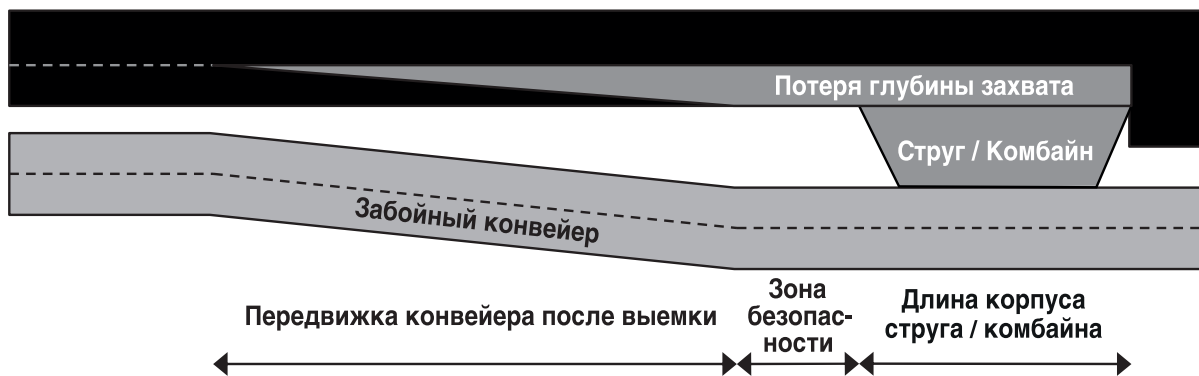
Рис. 6. Потери, обусловленные уменьшением глубины захвата
