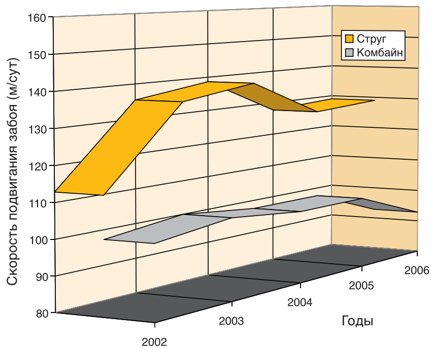
Рис. 8. Среднесуточное подвигание забоя в комбайновых и струговых лавах Германии 1
