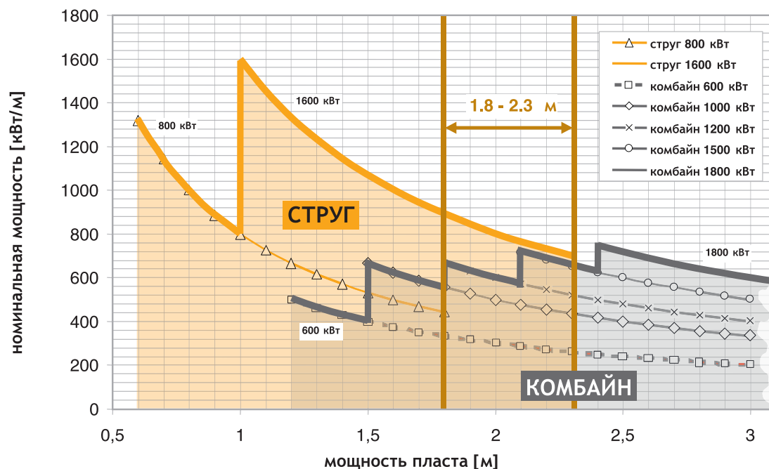
Рис. 14. Удельная мощность комбайна или струга в зависимости от высоты лавы
